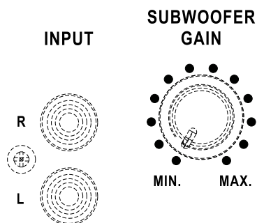
Figure 8 : connecteurs d'entrée du panneau arrière
